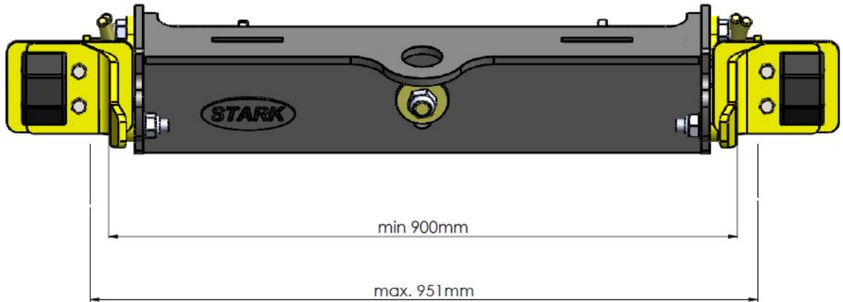
Kuva 1. Auraustuki.
